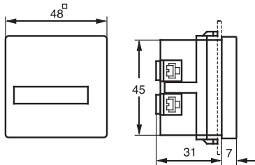
Montageausschnitt Quadrat: 48 x 48 mm Montageausschnitt Kreis: ø 50,5 mm
